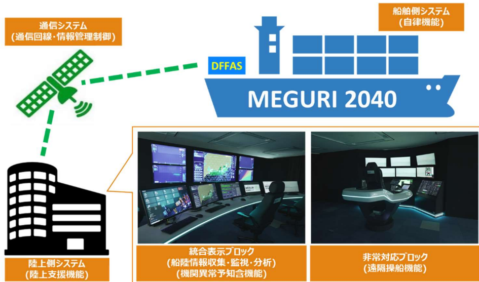
DFFAS コンソーシアムで開発した無人運航システムの概要 (陸上側システムから船舶の航行状況を監視し、有事には遠隔操船に切り替えも可能)
